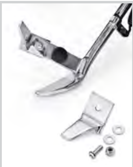
D. JIFFY STAND EXTENSION
