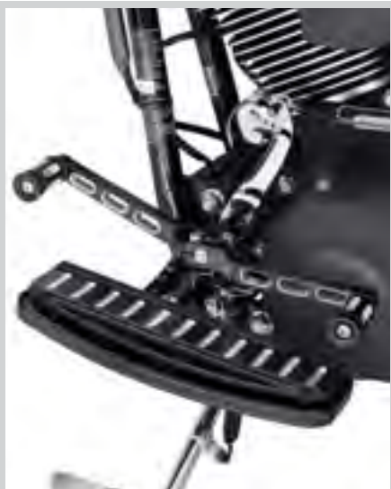
C. BILLET STYLE HEEL/TOE SHIFT LEVER – EDGE CUT
